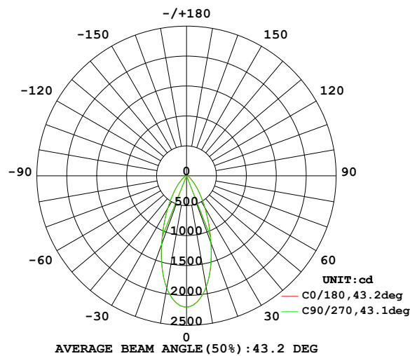
45° Beam Angle - 277V Input
