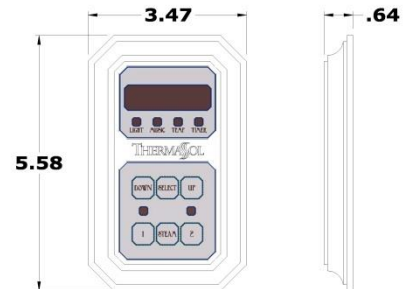
CONTROL BEZEL
