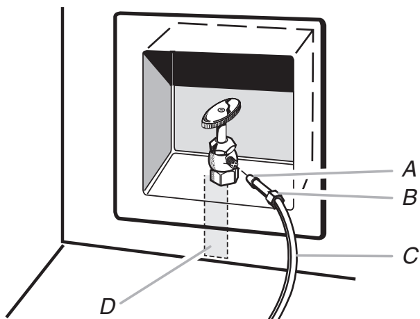
A. Manguito B. Tuerca C. Tubería de cobre (al refrigerador) D. Línea de suministro de la casa (1/2" (12,7 mm) como mínimo)
