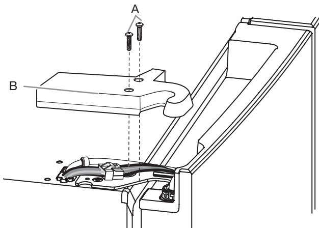
A. Vis du couvre-charnière supérieur
