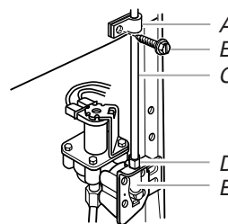
A. Bride du tube B. Vis de bride de tube C. Tube en cuivre D. Écrou de compression E. Valve d'entrée d'eau
