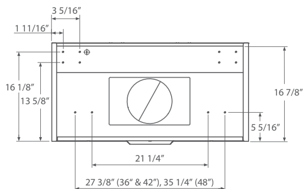
Arrière Dimensions d'installation
