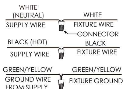
Fig. 4 Wiring guide
