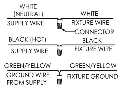
Fig. 4 Wiring guide
