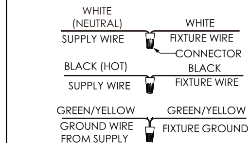
Fig. 4 Wiring guide
