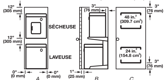
A. Encastrement B. Vue latérale - placard ou endroit exigu C. Porte de placard avec ouvertures d'entrée d'air
