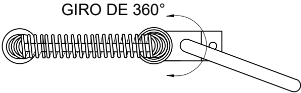
VISTA SUPERIOR
