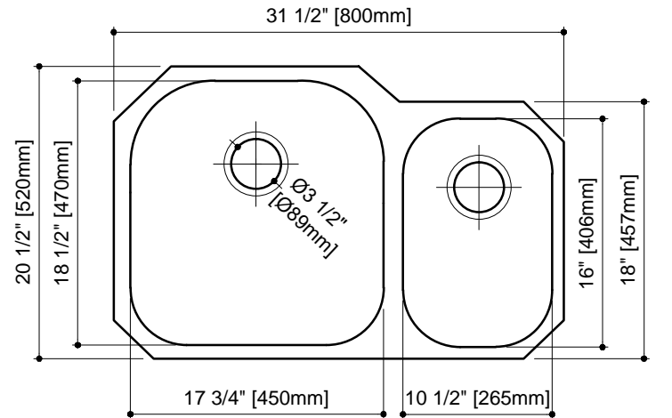
VISTA SUPERIOR
