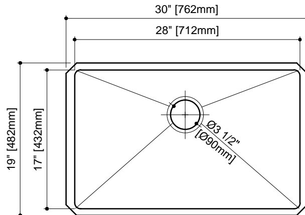
VISTA SUPERIOR
