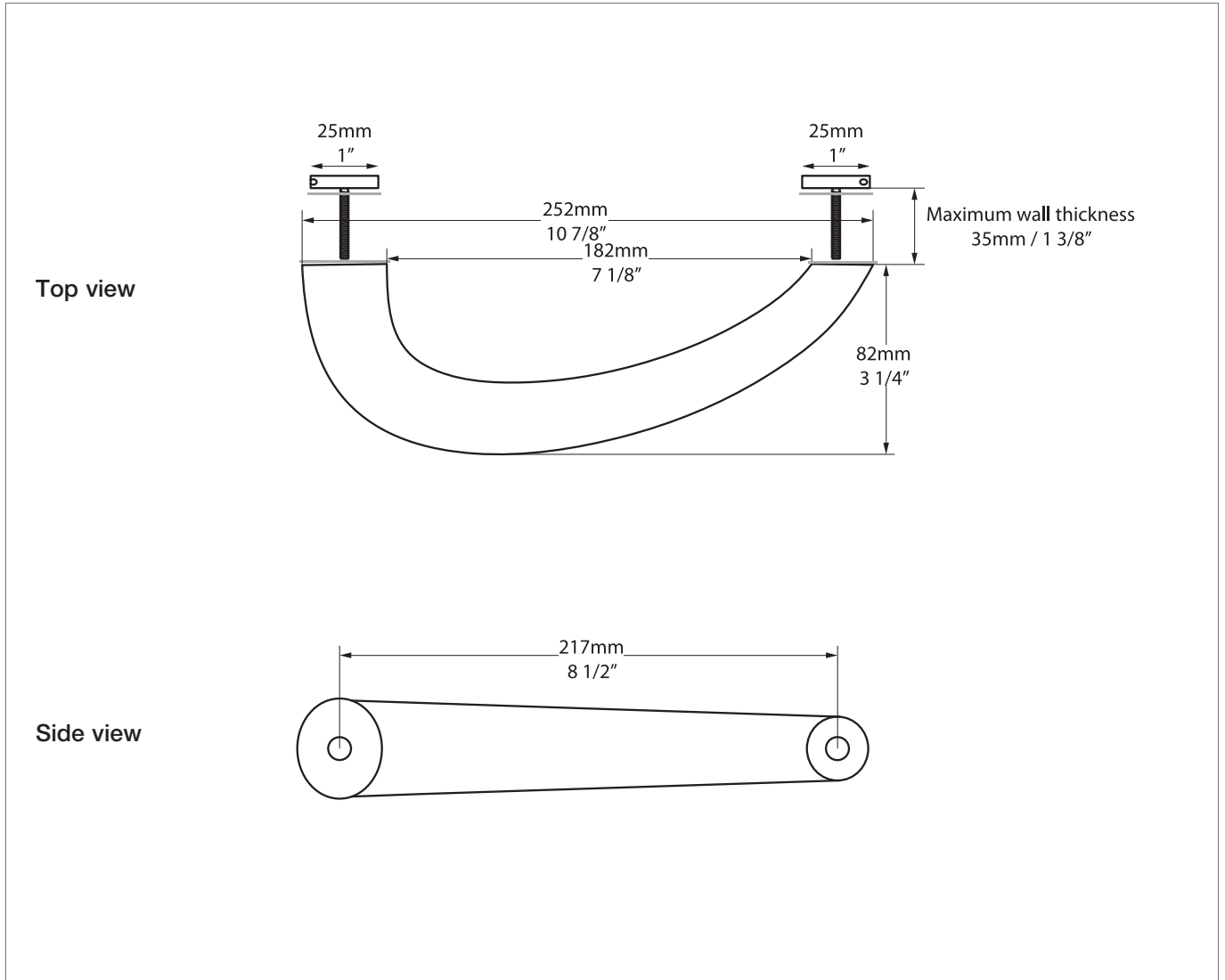
Set of two handles Lot de deux poignées Conjunto de dos asas
