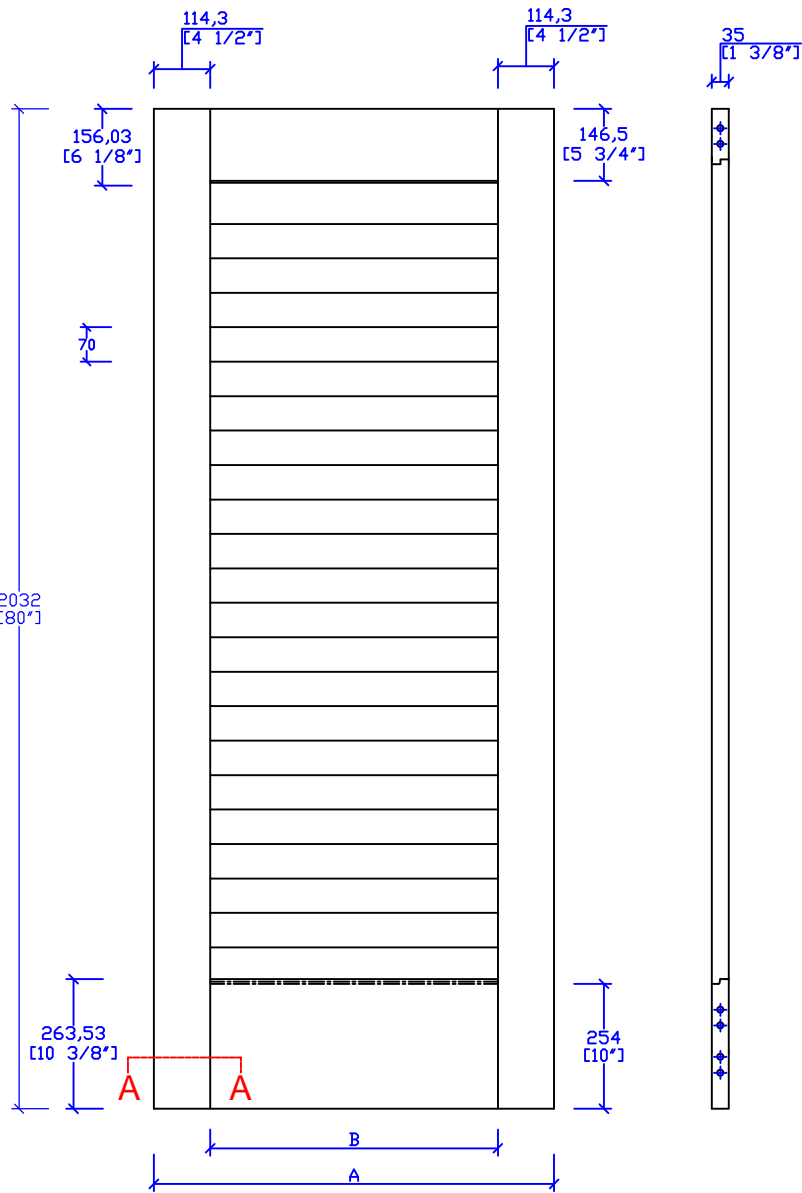
23 pcs Louver
