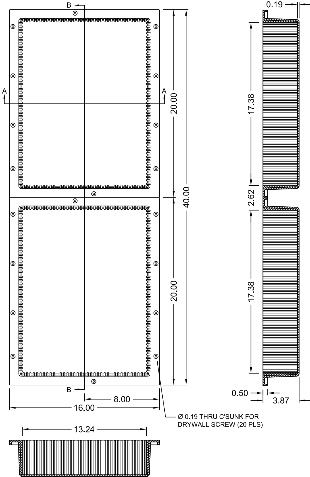
SECTION A-A
