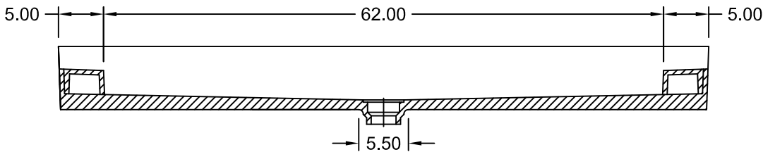
SECTION A-A
