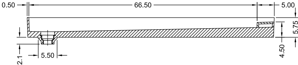
SECTION A-A
