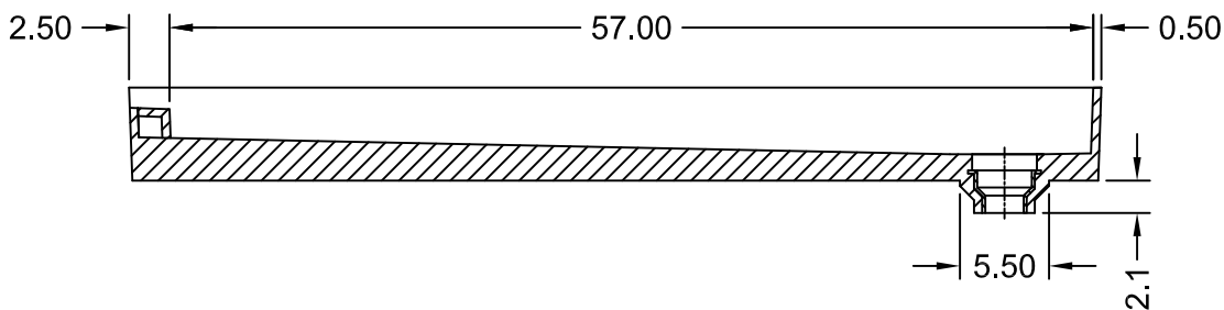
SECTION A-A
