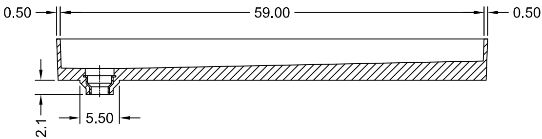
SECTION A-A
