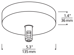
Mini Transformer
