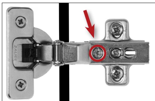
Adjusting door left & right
