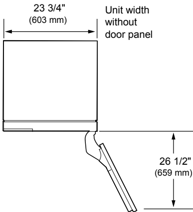
DOOR OPEN 115°
