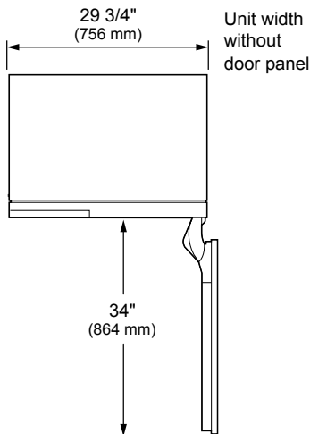
DOOR OPEN 90°
