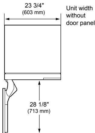
DOOR OPEN 90°
