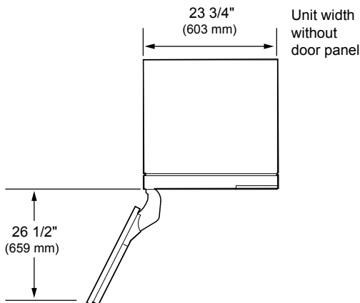
DOOR OPEN 115°
