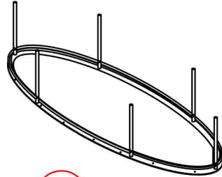
A1 * x1 Metal frame x1 Cadre en métal x1 Armazón de metal
