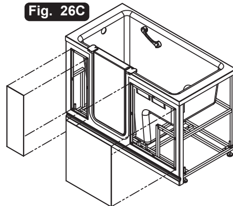
Ristorre™ 6030 ONLY
