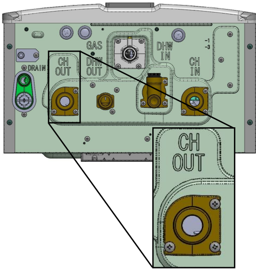
Raccord d'apport en chauffage
