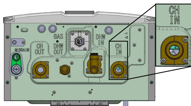
Raccord de retour de chauffage
