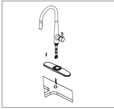
1. Installez le rosace sur le robinet. Insérez le nouveau robinet dans les trous prévus à cet effet sur le dessus du lavabo.
