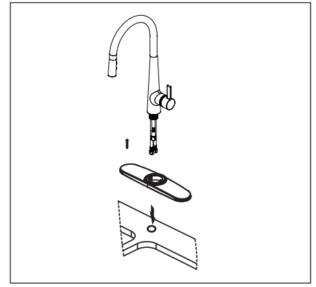
1. Instale la escudo sobre el grifo. Coloque el grifo nuevo a través de los orificios en la parte superior del lavabo.
