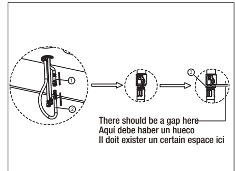
3. Conecte la manguera de salida (1) con la manguera desplegable (2). Confirme que el buje (3) vuelva a su estado original.
