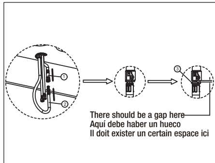
3. Branchez le flexible de sortie (1) au flexible rétractable (2). Vérifiez que le mamelon de raccordement conique (3) revient à sa position d'origine.
