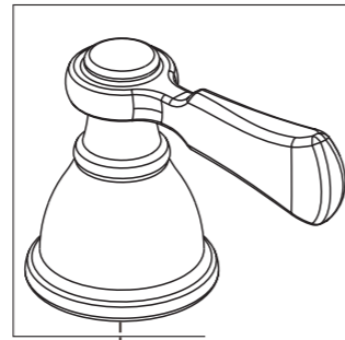
RP93981 Bonnet, Adapter & Valve Cartridge, Hot Side Bonete, Adaptador y Cartucho de la Válvula, Lado Chapeau, Adaptateur et Cartouche de soupape, Eau Chaude
