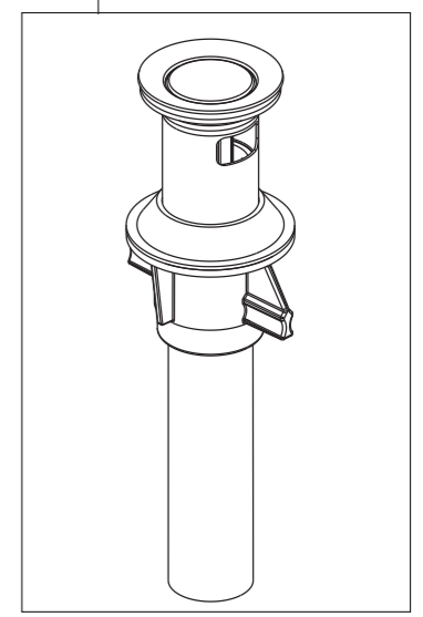
RP103419▲ 50/50 Push Pop-up Assembly Control de rebose para desagües manuales Renvoi mécanique à pousser avec trop-plein
