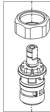
RP93981 Bonnet, Adapter & Valve Cartridge, Hot Side Bonete, Adaptador y Cartucho de la Válvula, Lado Chapeau, Adaptateur et Cartouche de soupape, Eau Chaude
