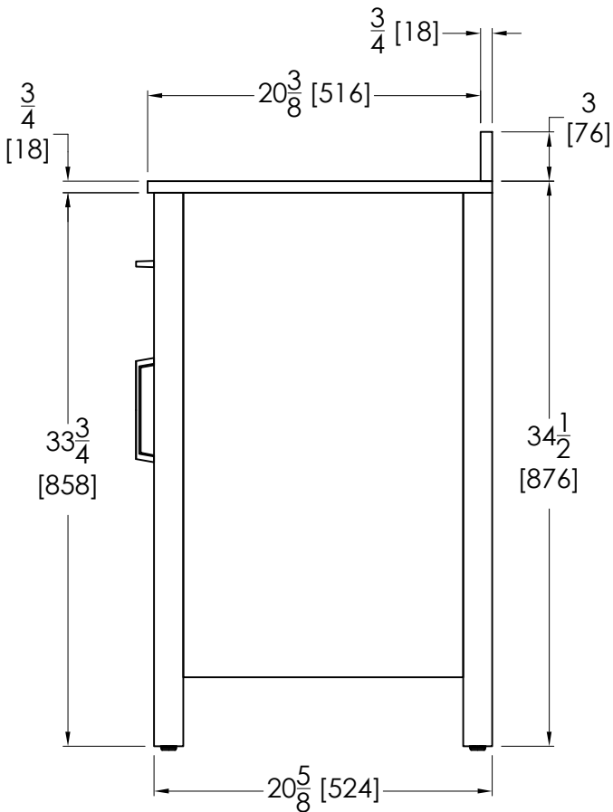
SIDE / CÔTÉ / LADO
