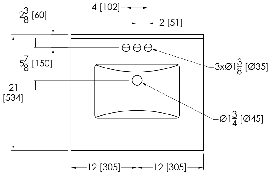
TOP / DESSUS / ARRIBA
