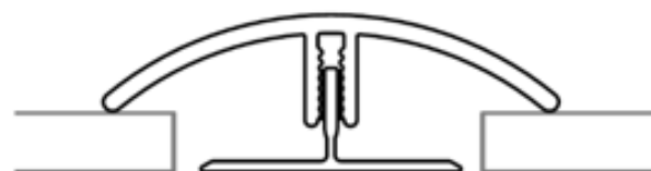
T-MOLDING
