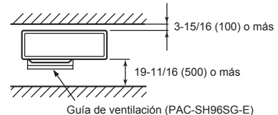
Guía de ventilación (PAC-SH96SG-E)
