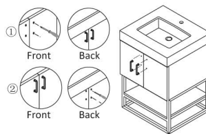
3. Install the handle/Installer la poignée
