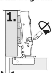
1. Side adjustment/ Ajustement du côté +0.08 -0.16
