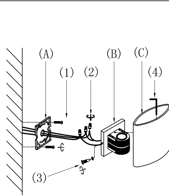
Back Plate/Plaque arrière (A)
