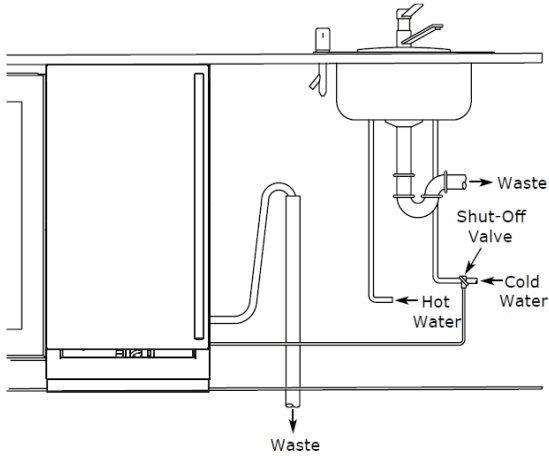
Stand Pipe
