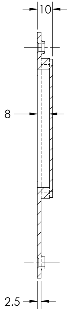
SECTION A-A
