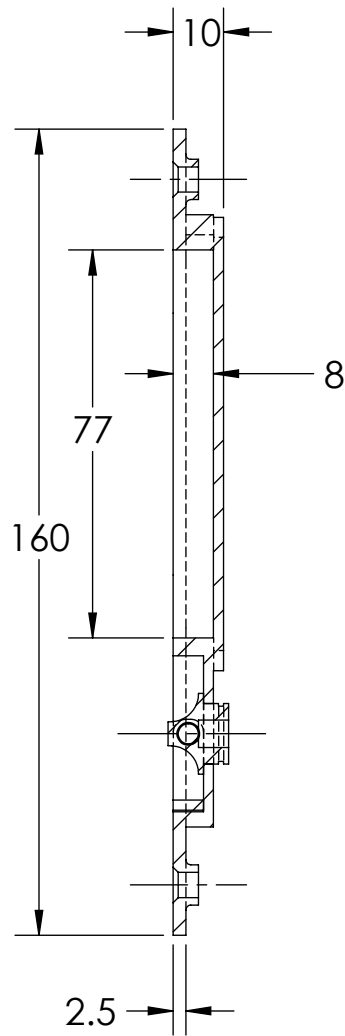
SECTION A-A
