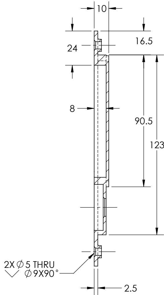
SECTION A-A SCALE 1 : 1.5
