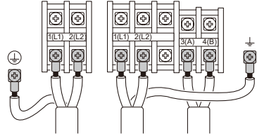
Câble d'alimentation électrique
