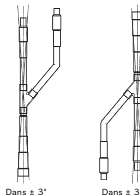
Configuration verticale vers le HAUT Configuration verticale vers le BAS
