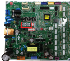
Carte à circuit imprimé principale (Maître)
