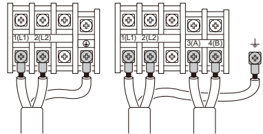
Câble d'alimentation électrique
