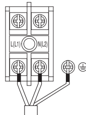
Cable de alimentación (208/230)
