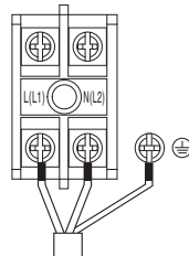
Cable de alimentación (208/230)
