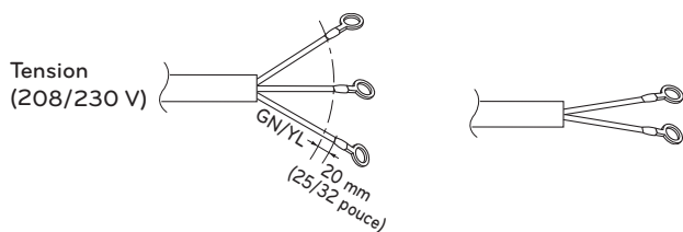
Cordon d'alimentation
