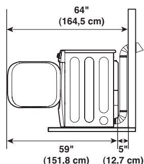
Conducto apto para instalación en pared .
