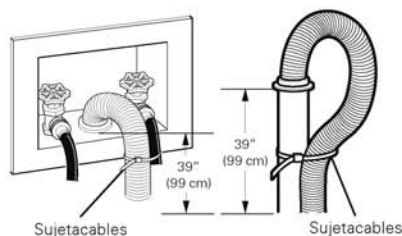
Sujetacables
