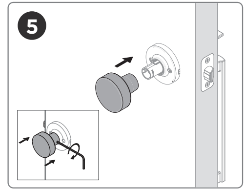
5 Reattach interior knob Vuelva a colocar la perilla interior Remettre le bouton intérieur en place
