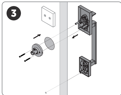
3 Secure together with mounting screws Fíjelo con los tornillos de montaje Fixer à l'aide des vis de montage
