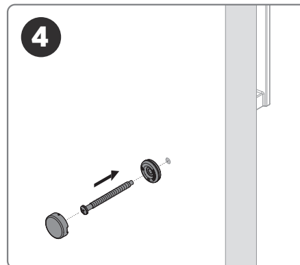
4 Secure bottom of handleset Asegure la parte inferior del jalador Fixez le bas de la serrure d'entrée à la poignée
