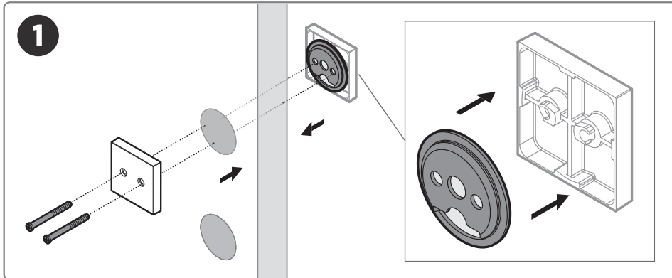
1 Install deadbolt Instalar cerrojo de seguridad Installer un verrou
