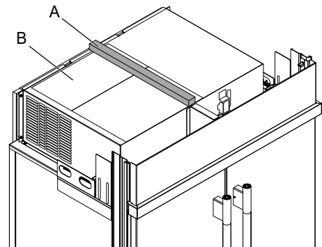
A. Joint d'étanchéité B. Couvercle du compresseur
