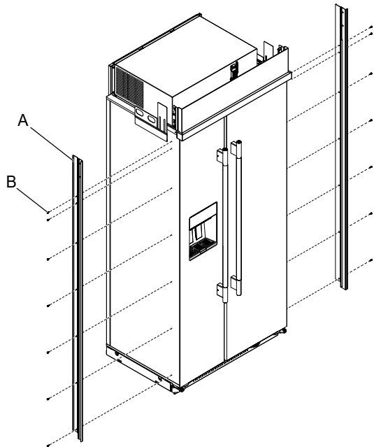
A. Molduras laterales B. Tornillos
