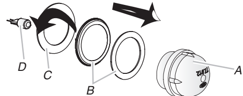
A. Glass cap B. Seals C. Metal ring D. Halogen bulb
