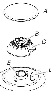
A. Chapeau de brûleur C. Base du brûleur B. Ouverture du tube d'arrivée de gaz D. Électrode d'allumage E. Porte-gicleur
