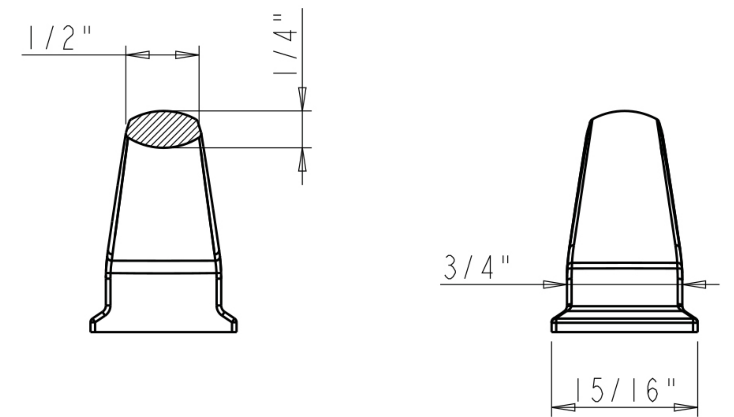
SECTION A-A
