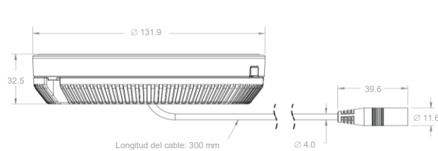
02. CARGADOR - VISTA DEL FRENTE
