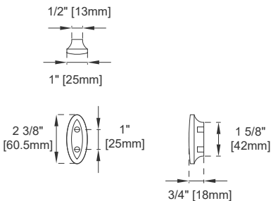
Knob
